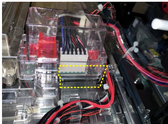
サブ中継基板ケースの下部、貼り付け範囲
