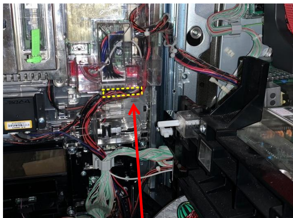
FGX-OU②取り付け位置 (サブ中継基板ケースの下部)
